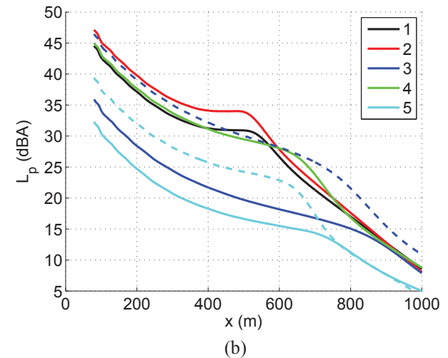
FIGURE 7 – Niveau de pression L_p en dB(A) en fonction de x pour z = 1, 5 m (a) pour les atmosphères 1 (traits continus) et 6 (traits tirets) et pour différents angles de propagation \theta , et (b) pour \theta = 180^\circ pour toutes les atmosphères (traits continus pour les profils théoriques et traits tirets pour les profils mesurés).
