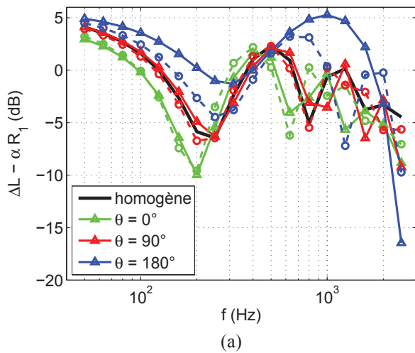
FIGURE 5 – Spectres en tiers d'octave de \Delta L - \alpha R_1 pour les atmosphères 1 (triangles) et 4 (cercles) et pour différents angles de propagation \theta en z = 1, 5 m et en (a) x = 500 m et (b) x = 1000 m.
