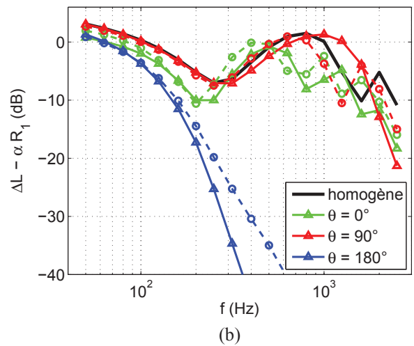
FIGURE 5 – Spectres en tiers d'octave de \Delta L - \alpha R_1 pour les atmosphères 1 (triangles) et 4 (cercles) et pour différents angles de propagation \theta en z = 1, 5 m et en (a) x = 500 m et (b) x = 1000 m.
