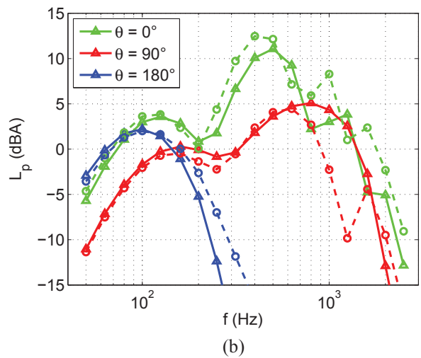
FIGURE 6 – Spectres en tiers d'octave du niveau de pression en dB(A) pour les atmosphères 1 (triangles) et 6 (cercles) et pour différents angles de propagation \theta en z = 1, 5 m et en (a) x = 500 m et (b) x = 1000 m.
